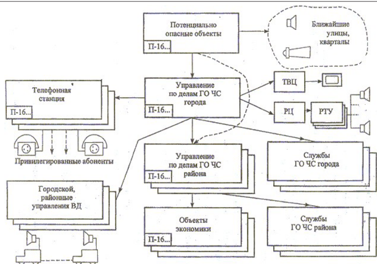
Рисунок 2 – Организация системы оповещения города
