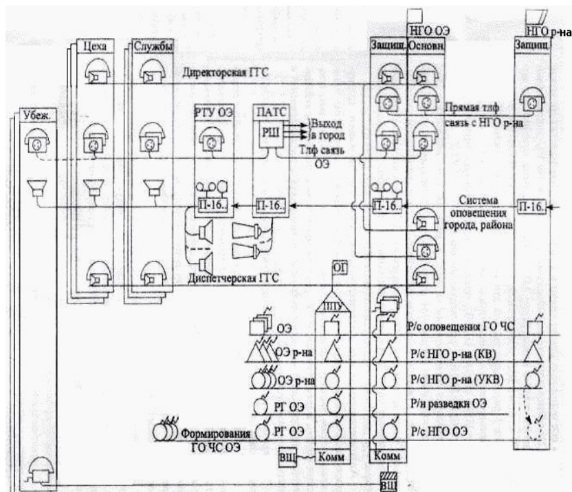
Рисунок 1 – Схема оповещения связи и оповещения ОЭ (вариант)
