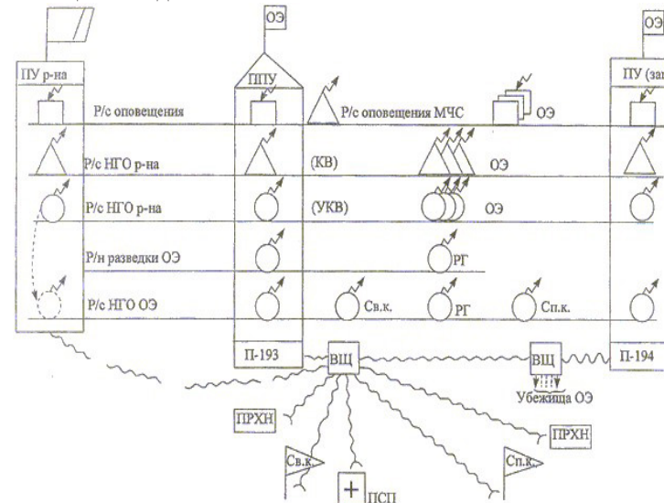
Рисунок 3 – Организация связи в очаге поражения
