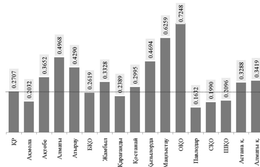
Сурет 1 – Өңірлердің 2011 жылғы қауіпсіздік деңгейлері
